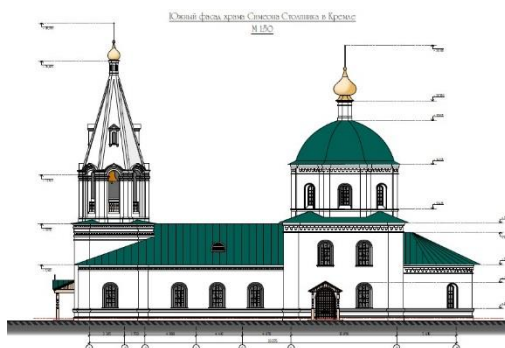
Рис. 3а. Проект восстановления церкви 2019 г. – на первую половину XIX в.
