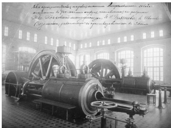
Рис. 5. Интерьер электростанции отделочного корпуса Товарищества Покровской мануфактуры П. Н. Грязнова в г. Иваново-Вознесенске. ГАИО. Публикуется впервые
