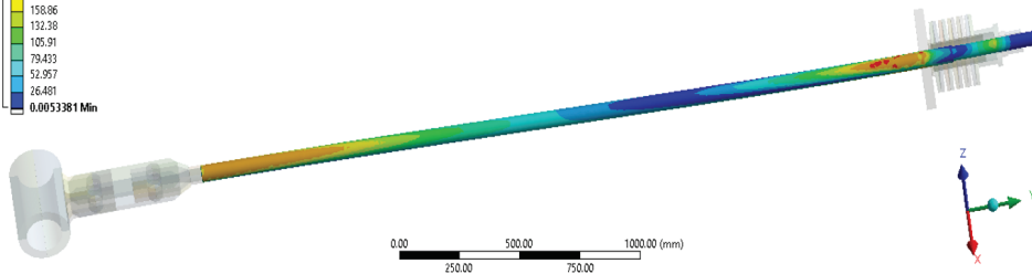
Рис. 5. Напряжения в наиболее нагруженной тяге подвески по результатам расчетов в ANSYS на основании данных о перемещениях и усилиях из SCAD Office
