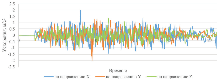
Рис. 3. Синтезированные акселерограммы
