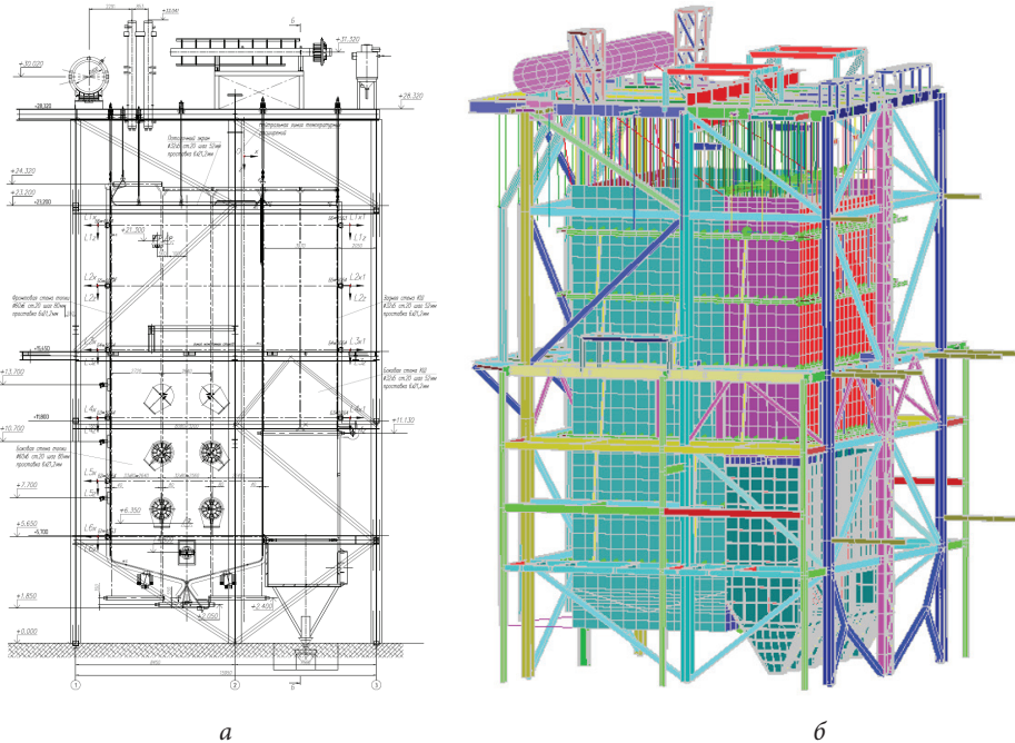
Рис. 1. Рассматриваемая система «каркас – котел»: а – установочный чертеж парового котла и каркаса; б – расчетная схема системы «каркас – котел» в SCAD Office
