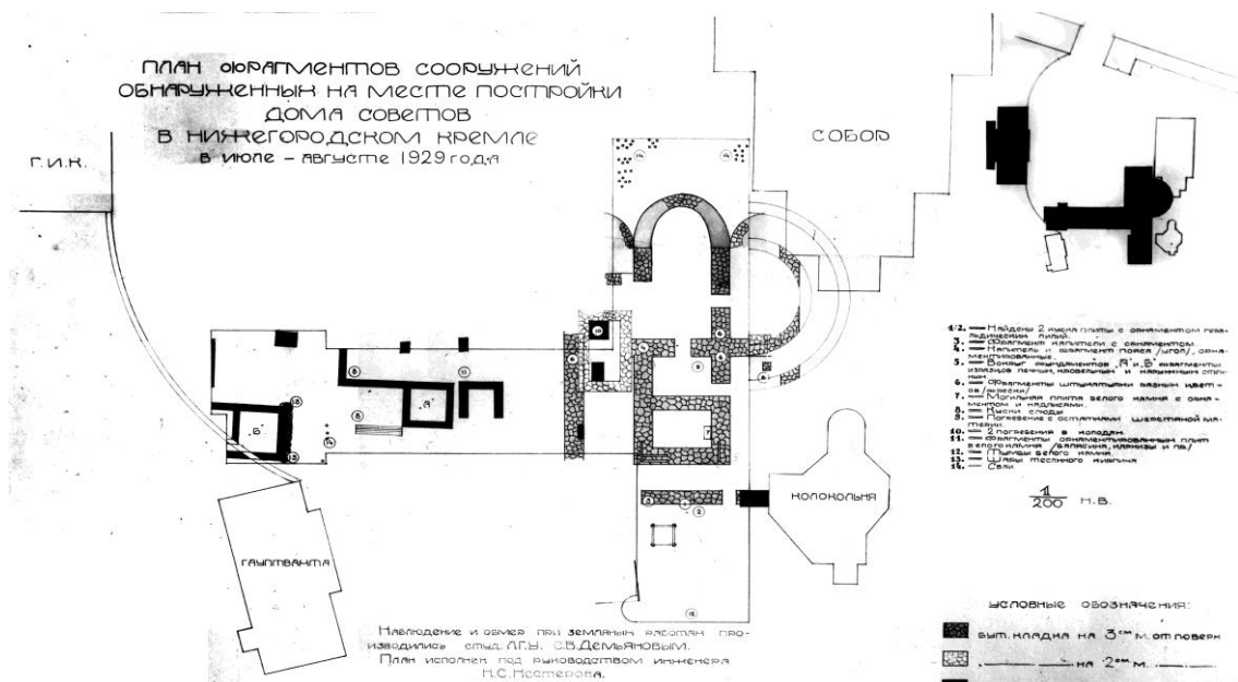
Рис. 2. План участка кремля с указанием взаиморасположения Спасо-Преображенского собора, колокольни и возводимого Дома Советов. Обмерный чертеж 1929 г. выполнили С. В. Демьянов и Н. С. Нестеров. В границах плана Дома Советов показаны фундаменты старого собора и других исторических построек. Архивный чертеж
